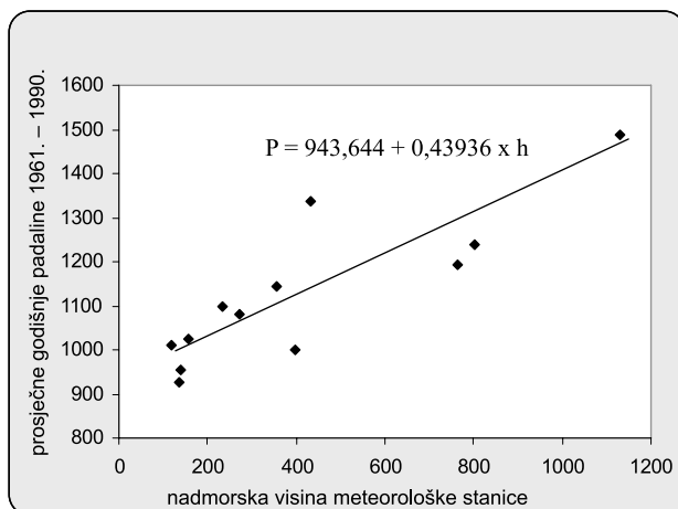
Sl. 4.: Pravac regresije odnosa nadmorske visine i prosječne godišnje količine padalina za odabrane stanice šire istraživnog područja (isključujući Mlinište)
