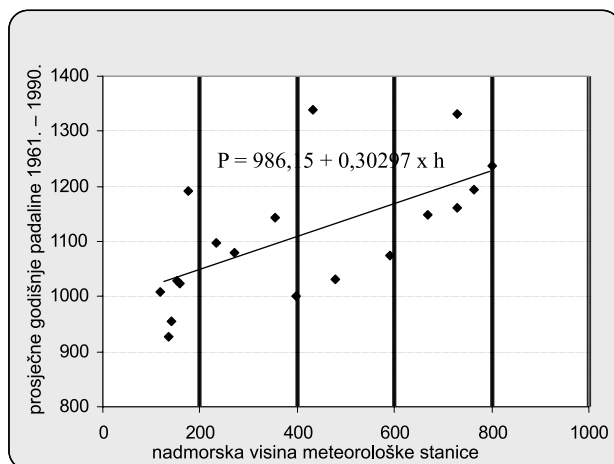
Sl. 3.: Pravac regresije odnosa nadmorske visine i prosječne godišnje količine padalina za odabrane stanice šire istraživnog područja (isključujući Mlinište)
