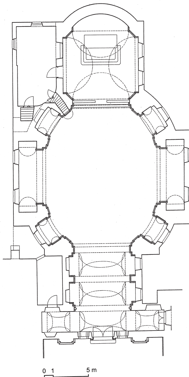
Maribor, Isusovačka crkva sv. Alojzija, tlocrt (arhitektonska snimka: D. Stepinac)
