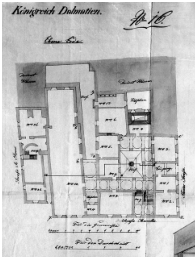
Tloct prizemlja crkve Sv. Petra Starog i Andrije, Sv. Marcele i istoimenog samostana, 1828. g.
