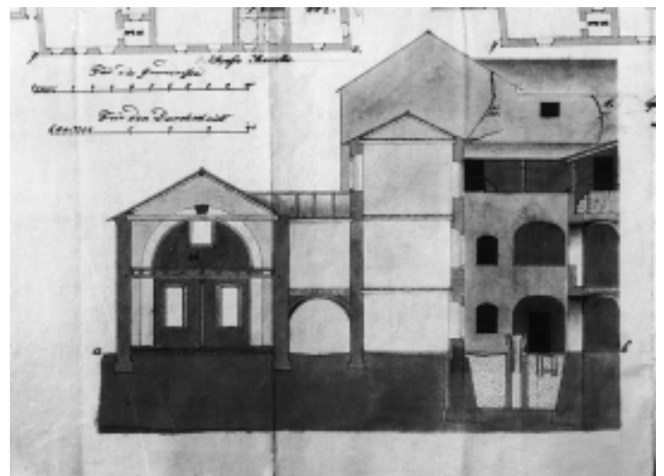
Poprečni presjek kroz crkvu i samostan Sv. Marcele, 1828. g.
