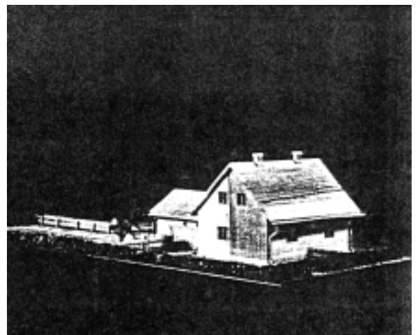
Maketa radničke kuće u naselju »Ante Starčevića« u Donjoj Dubravi (»Hrvatski narod«, 27. VI. 1941)
