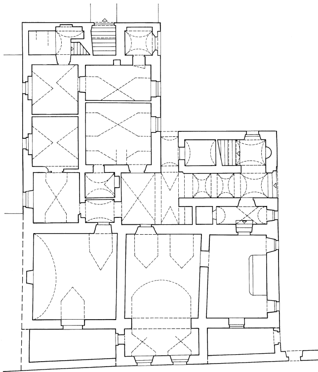
Prizemlje
