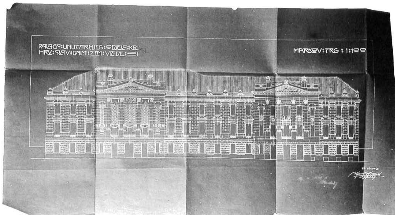
Nacrt pročelja sabornice na Markovu trgu, Janko Kolarić, 1907. godina (Povijesni arhiv Zagreb) Plan of the front of the Assembly building on St. Mark's Square, Janko Kolarić, 1907
