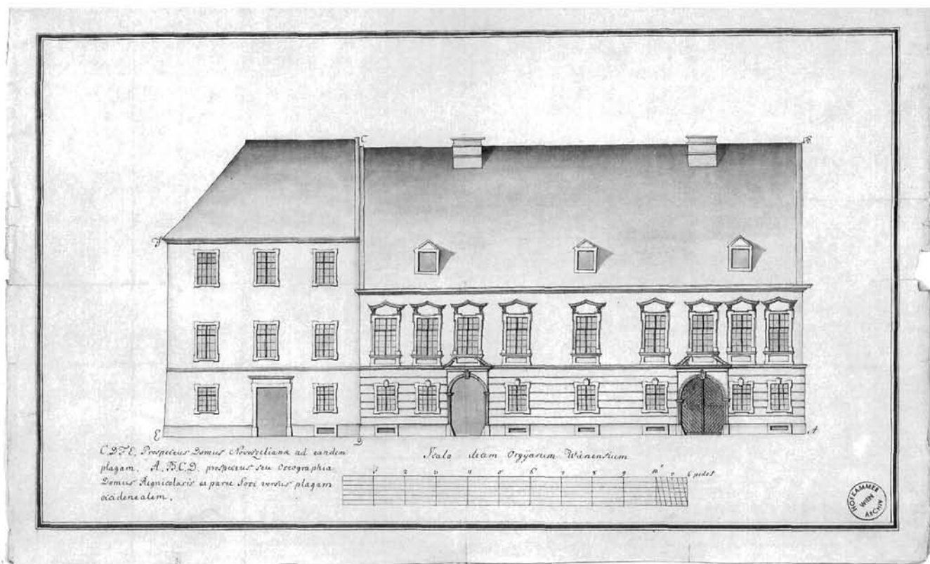
Pročelje saborske palače, 1770. godine (Hofkammerarchiv, Beč) Front elevation of the Assembly building, 1770
