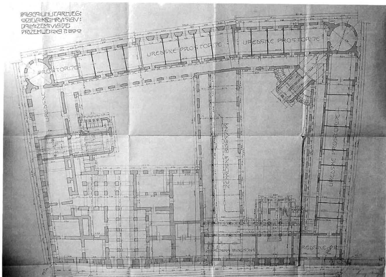
Sabor'ska palača prema projektu Aleksandra Brdarića, uklopljena u projekt kompleksa tzv. Vladine palače, 1908. godine, tlocrt (Povijesni arhiv Zagreb)
