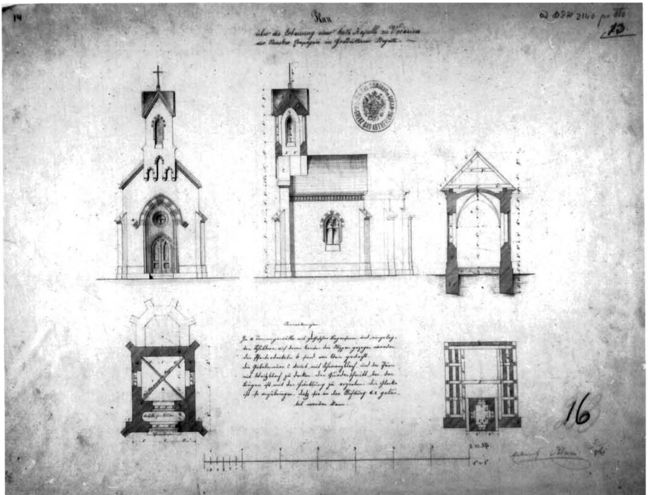
F. Klein: Načrt za katoličku kapelu u Voćarici (1861.) (Dijeccezanski muzej Zagreb) F. Klein: Sketch for a Catholic chapel in Voćarica (1861). Diocesan Museum, Zagreb
