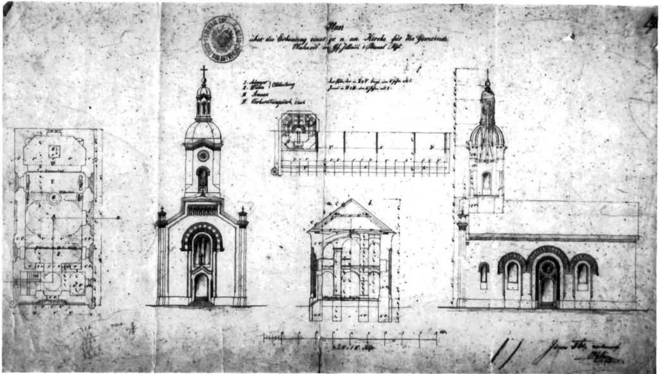
F. Klein: Načrt za pravoslavnu crkvu u Vlahoviću (1861.). (Dijecezanski muzej Zagreb) F. Klein: Design for an Orthodox church in Vlahović (1861). Diocesan Museum, Zagreb
