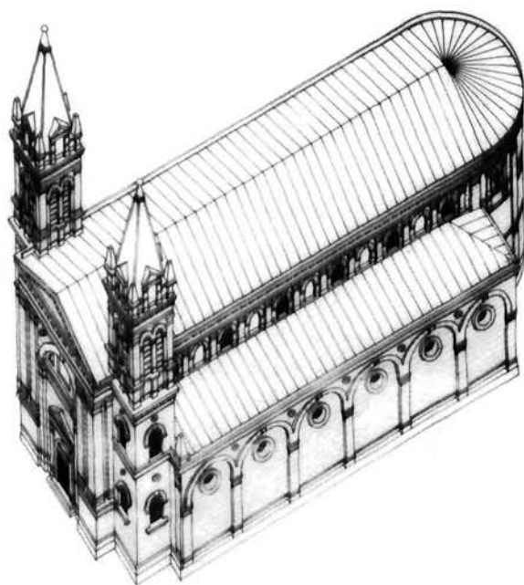
Zlatko Jurić, aksonometrija prema projektu J. Vančaša za crkvu sv. Blaža, 2. 12. 1891. (foto: I. Buzjak) Zlatko Jurić, axonometric drawing of J. Vančaš's design for the Church of St. Blaise, 2. 12. 1891.
