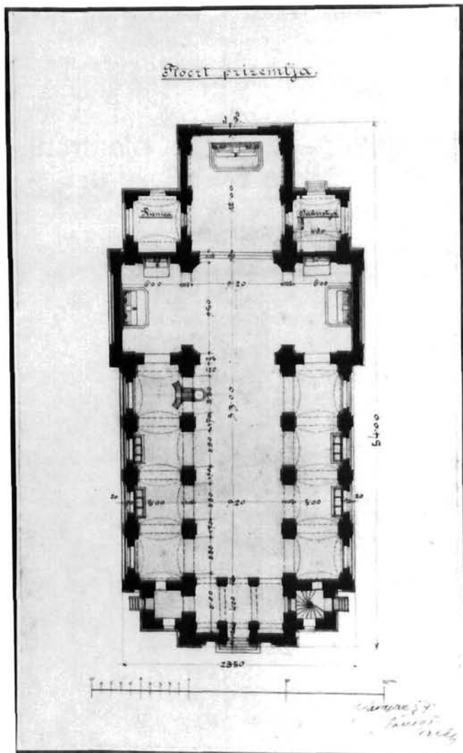
Josip Vančaš, tlocrt prizemlja crkve sv. Blaža. 5. 8. 1891. (KAZ; foto: I. Buzjak) Josip Vančaš, ground plan of the Church of St. Blaise, 5. 8. 1891.
