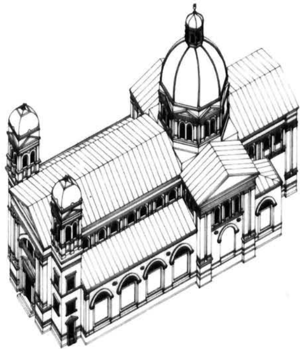
Zlatko Jurić, aksonometrija prema projektu J. Vančaša za crkvu sv. Blaža od 3. 8. 1891. (foto: I. Buzjak) Zlatko Jurić, axonometric drawing based on Josip Vančaš's design for the Church of St. Blaise, 3. 8. 1891.
