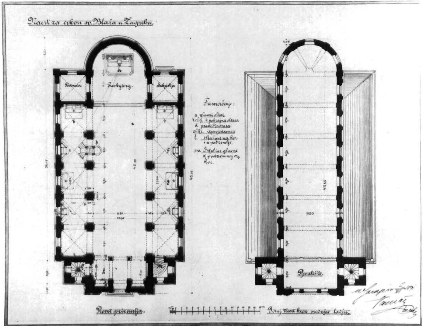
Josip Vančaš, tlocrt prizemlja i gornji tlocrt srednjega broda, 2. 12. 1891. (KAZ; foto: I. Buzjak) Josip Vančaš, plan of the ground floor and upper ground plan through the central nave, 2. 12. 1891.
