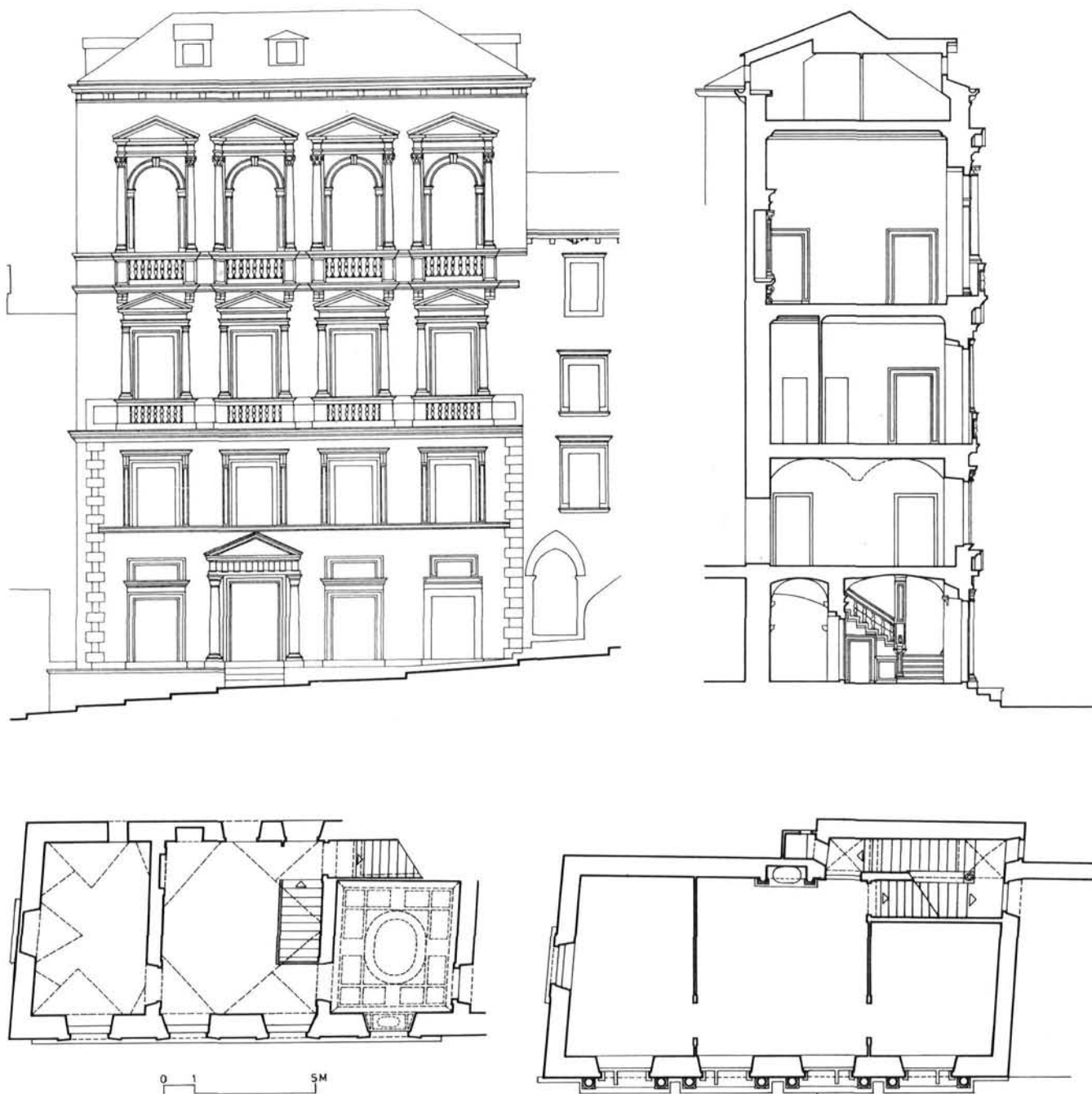
Palača Skočibuha u Restičevoj ulici 1, tlocrti prvog i trećeg kata pročelje i presjek
