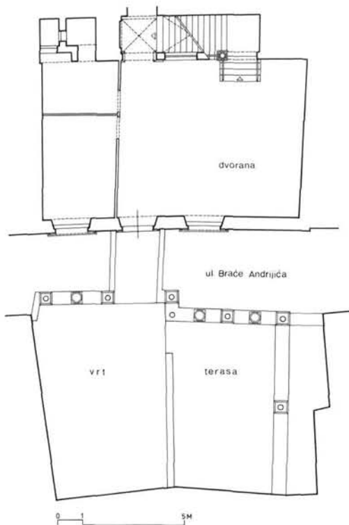
Barokna palača u Ulici braće Andrijića 8: tlocrt prvoga kata stambenoga dijela, vrta i terase (prijedlog rekonstrukcije)
