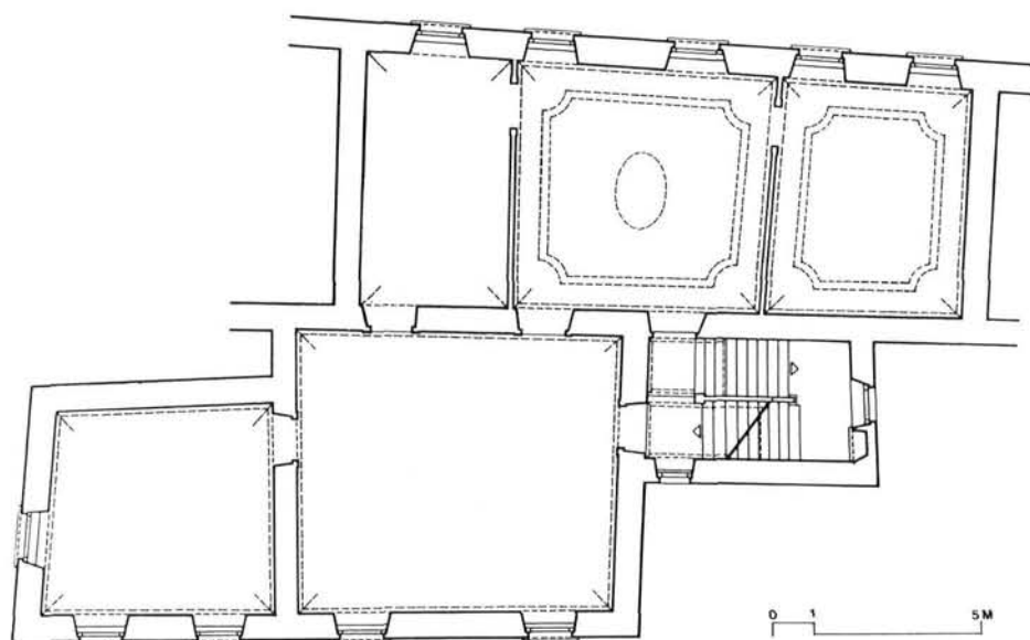
Karakteristični tlocrti baroknih palača u Ulici braće Andrijića 2 i 1 (palača Sorkočevića), prijedlog rekonstrukcije
