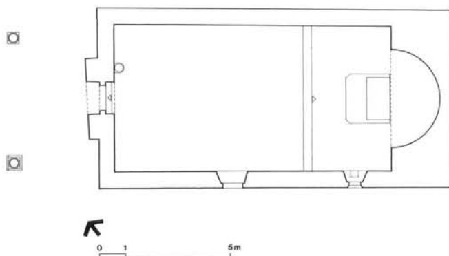
Hum, kapela sv. Jeronima, tlocrt
