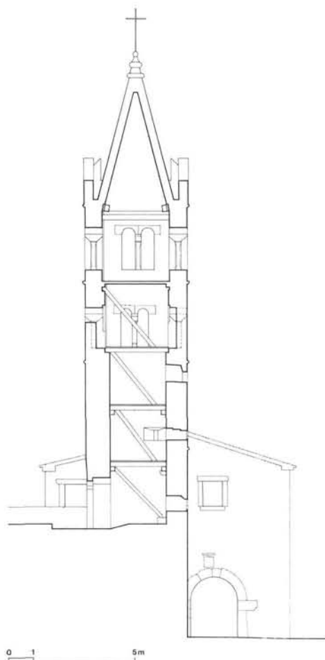
Hum, presjek kroz zvonik-kulu s pogledom na Glavna gradska vrata
