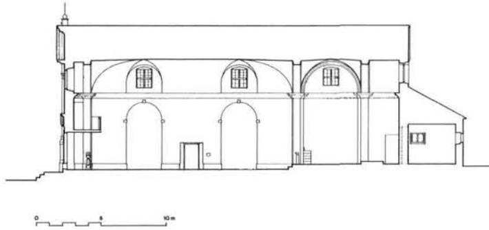
Hum, župna crkva sv. Marije, uzdužni presjek
