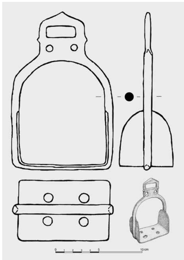
sl. 2. Ranosrednjovjekovni stremen iz Pliske u Bugarskoj (crteži: N. Šimundić Bendić).
