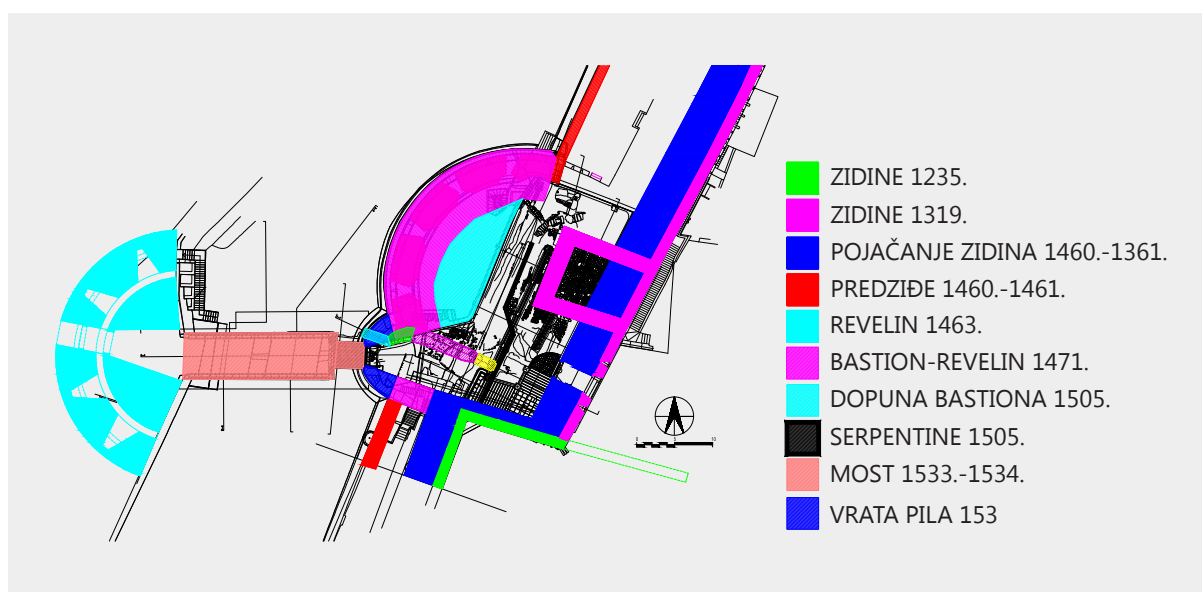
sl. 24. Pile u prvoj polovini 16. stoljeća (tlocrt: Ž. Peković).
