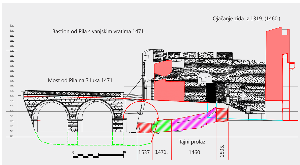
sl. 18. Pile u 15. stoljeću (presjek: Ž. Peković).
