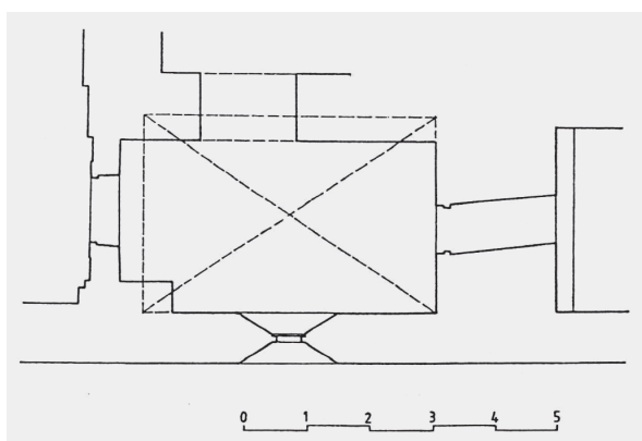
sl. 5. Tlocrt prizemlja zvonika male braće u Dubrovniku (Ž. Peković, 1991.).
