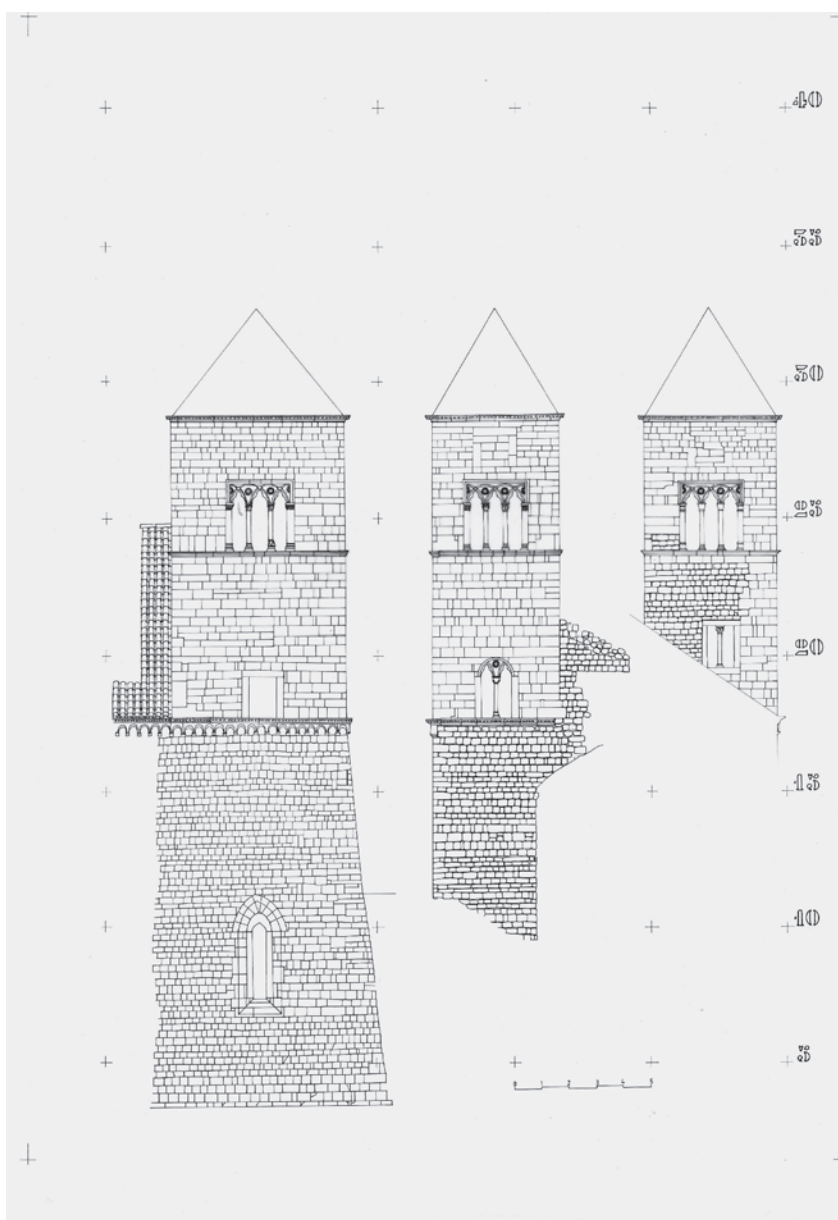
sl. 6. Rekonstrukcija prve faze zvonika male braće u Dubrovniku (Ž. Peković, 1991.).
