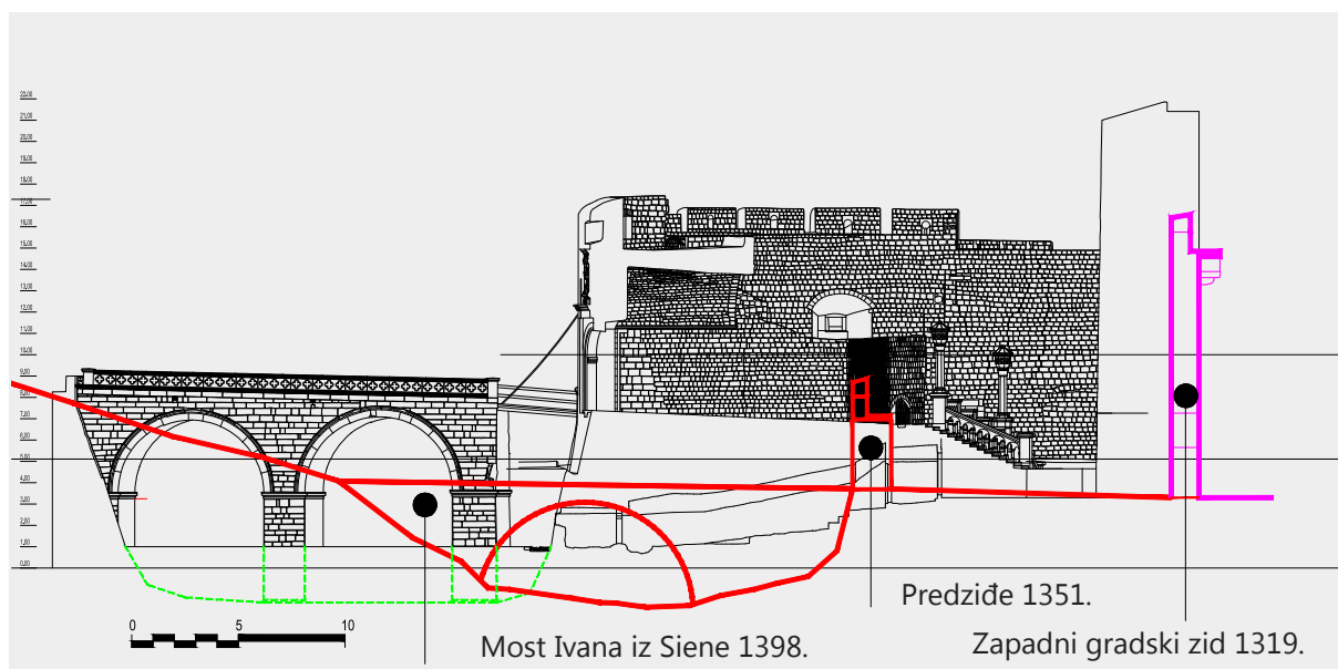
sl. 15. Pile u drugoj polovini 14. stoljeća (presjek: Ž. Peković).
