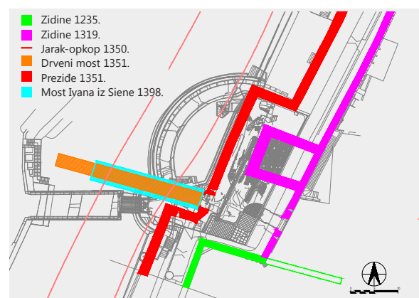
sl. 13. Pile u drugoj polovini 14. stoljeća (tlocrt: Ž. Peković).
