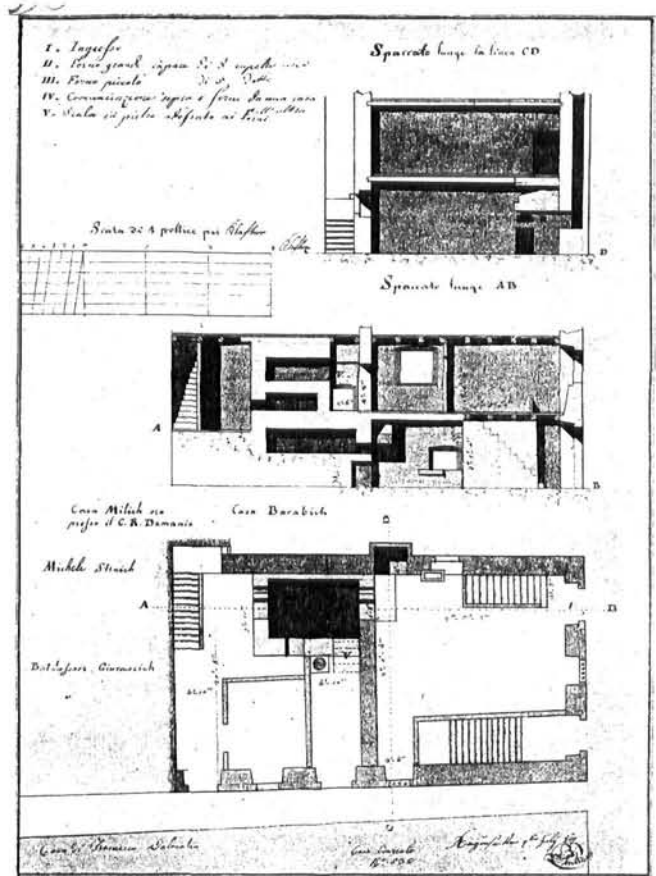
Presjek kuće Nikole Učovića (arhitekt Boriani, 1817. godine)
