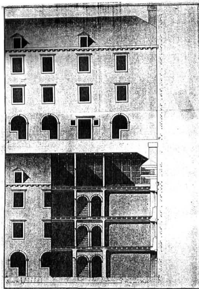
Pročelje i presjek kuće Mihovila Čuklića (arhitekt Boriani, 1817. godine)
