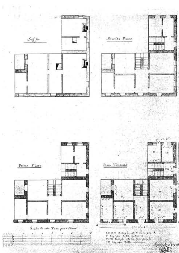
Plan za novogradnju pekare u kući Nikole Učovića (arhitekt Boriani, 1817. godine)
