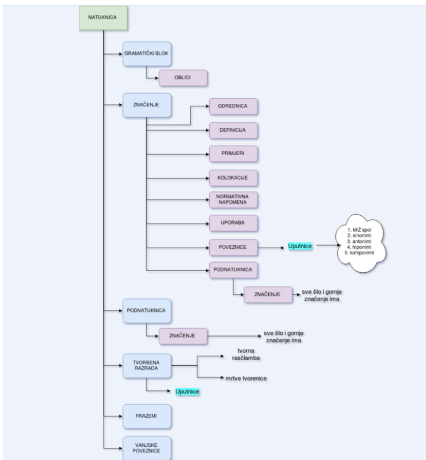
Slika 2. Struktura rječničkoga članka u osnovnome modulu Mrežnika
