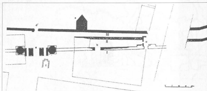
Sl. 22.: Bedemi Zadra s kopnene strane. I – ranoantički bedem; a – Bersin slavluk, b – Porta Media, c – vrata s kulama kvadratne osnove; II – kasnoantički bedem; III – srednjovjekovni bedem (preuzeto iz: GIUNIO 2001., sl. 23.)
