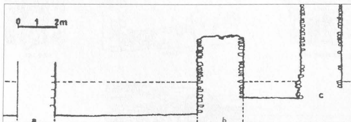
Sl. 23.: Nivelete bedema Zadra s kopnene strane. a – ranoantički bedem; b – kasnoantički bedem; c – srednjovjekovni bedem. (preuzeto iz: GIUNIO 2001., sl. 24.)
