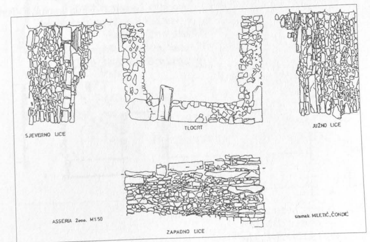
Sl. 20.: Tlocrt i bokocrti kasnoantičke kule u Aseriji (preuzeto iz: FADIĆ 2001., sl. 13.)
