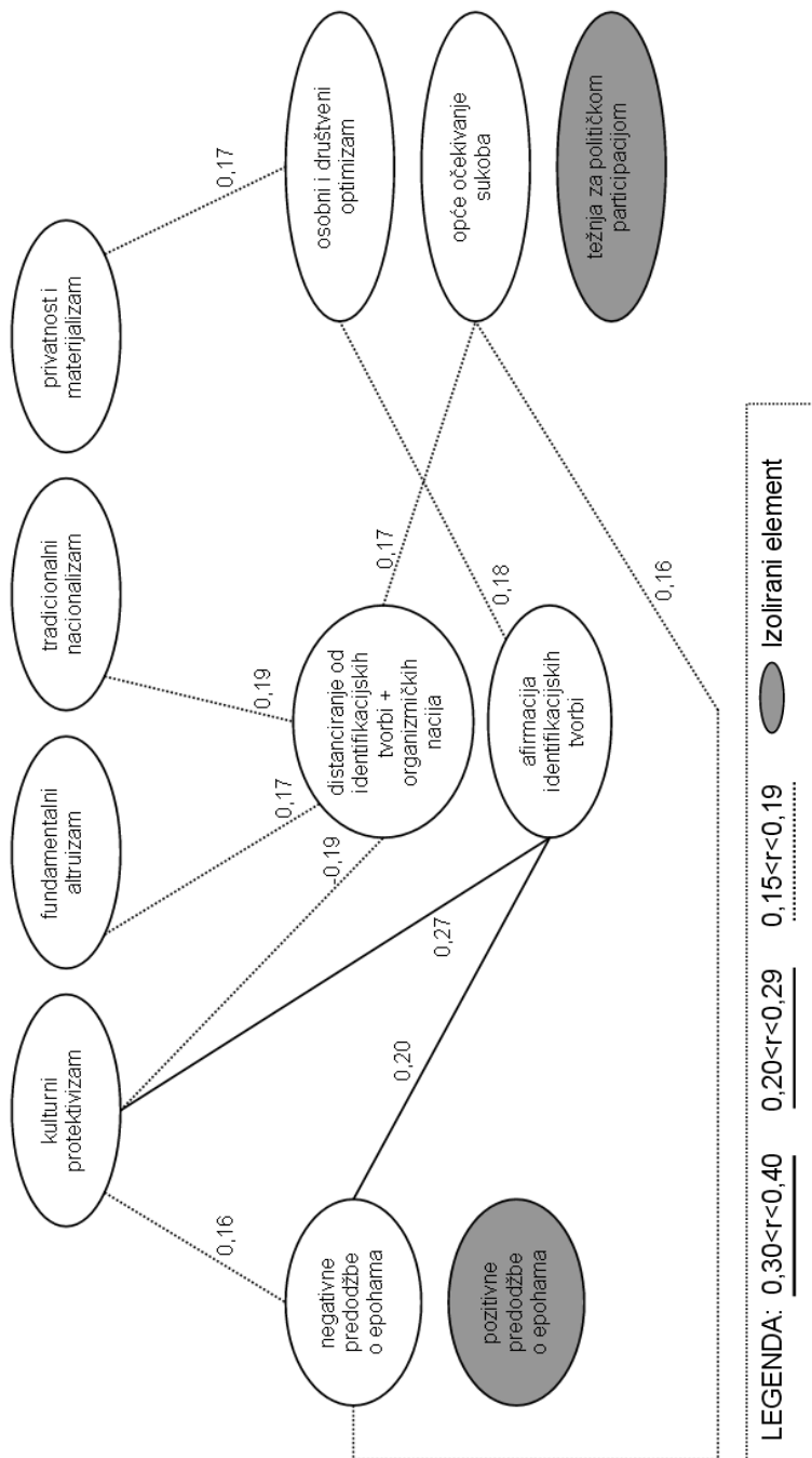
Slika 7. Parcijalne povezanosti općih čimbenika povijesne svijesti u Istočnoj Europi.
