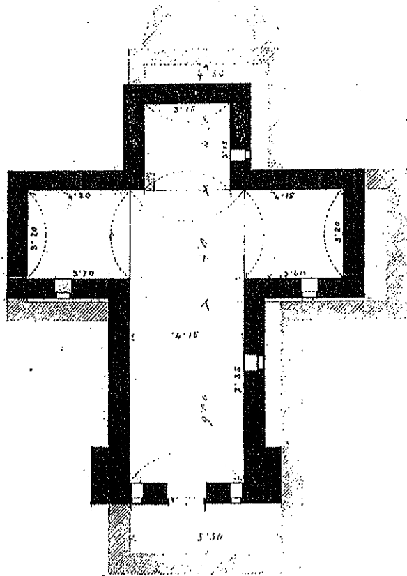
Tloris župne crkve u Bogomolju iz 1835. (PAZd, Građevinska sekcija, br. 149)
