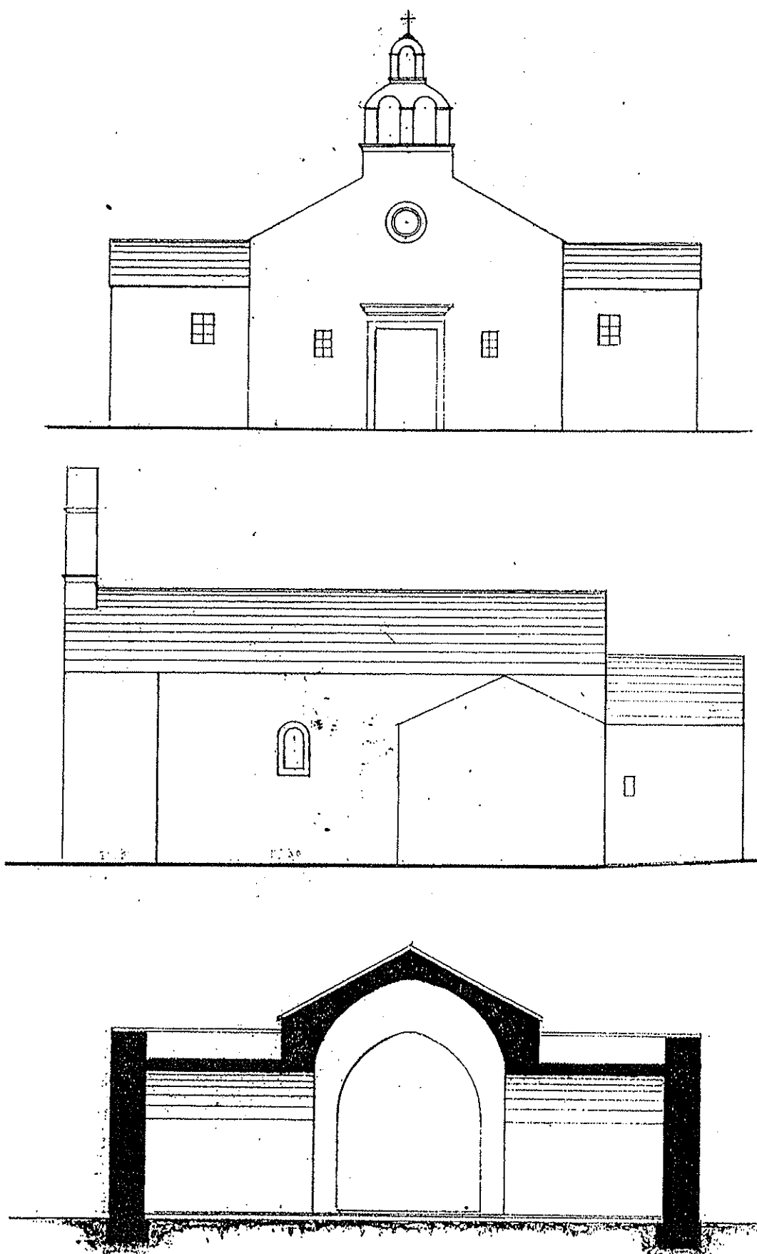
Arhitektonski snimak župne crkve u Bogomolju 1885. g. (PAZd, Građevinska sekcija br. 149)
