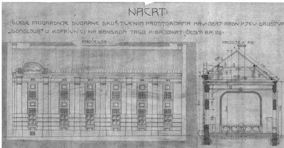
Sl. 3. Pročelje »Domoljuba« prema nacrtu iz lipnja 1919. godine u mjerilu 1:200 (izvor: Muzej grada Koprivnice)
