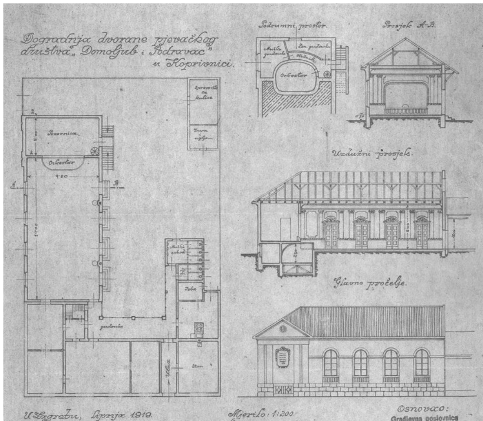
Sl. 2. Tlocrtni nacrt i presjeci dvorane »Domoljub« iz lipnja 1919. godine u mjerilu 1:200 (izvor: Muzej grada Koprivnice)
