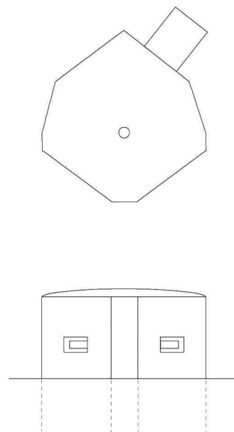
Peterokutni bunker Pogled odozgo i sa strana MJ. 1:50
