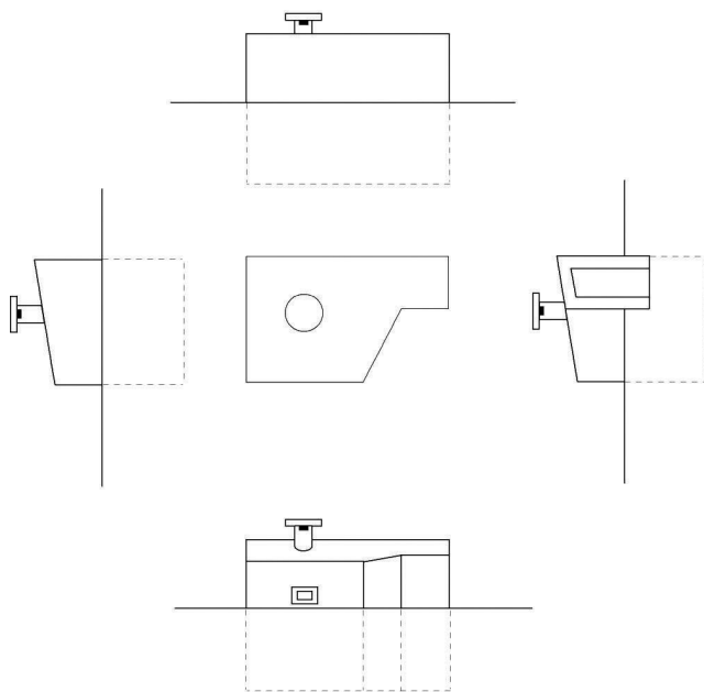
Karakteristican bunker Pogled odozgo i sa strana MJ. 1:50
