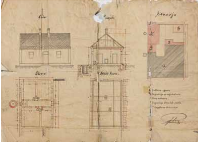
Nacrt zatvora iz oko 1903. g. (Muzej grada Koprivnice)
