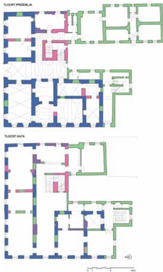
Tlocrt prizemlja i kata. Razvojne faze. 1. faza (17. ili prva polovica 18. st.) – plava boja, 2. faza (18. st.) – crvena boja, 3. i 4. faza (19. i 20. st.) – zelena boja. (Hrvatski restauratorski zavod)
