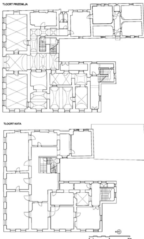
Predložena rekonstrukcija. Tlocrt prizemlja i kata. (Hrvatski restauratorski zavod)
