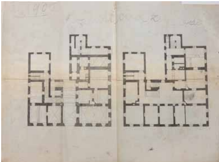
Nacrt zgrade iz 1905. g. (Muzej grada Koprivnice)
