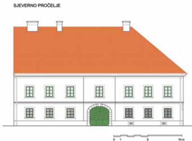
Glavno pročelje. Predložena rekonstrukcija
