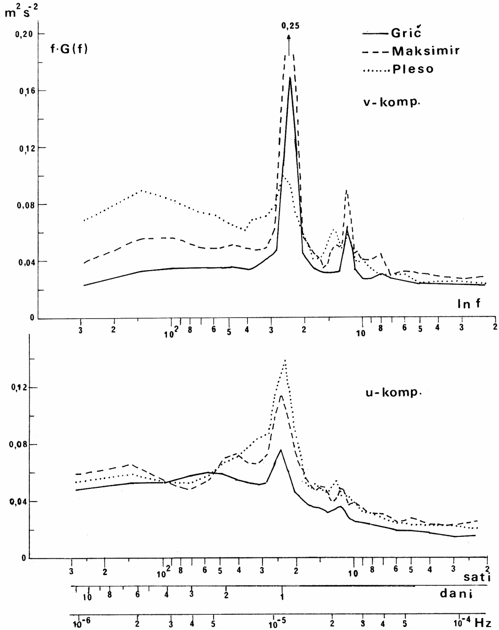
Slika 31. Godišnji spektri energije zonalne i meridionalne komponente vjetra za tri postaje šireg područja Zagreba, prema satnim vrijednostima (Grič 1956–60, Maksimir i Pleso 1969).
