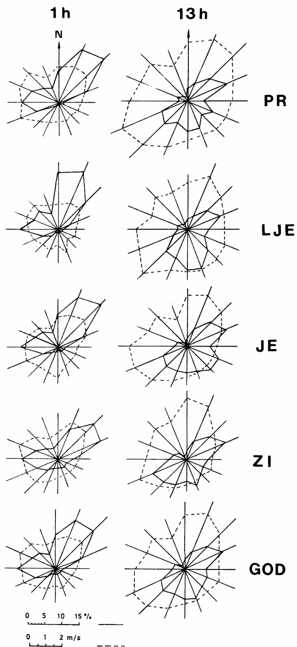
Slika 5. Sezonske i godišnja ruža smjera i brzine vjetra prema satnim vrijednostima u 1 i 13 h na anemogramu, Zagreb–Grič 1951–60.
