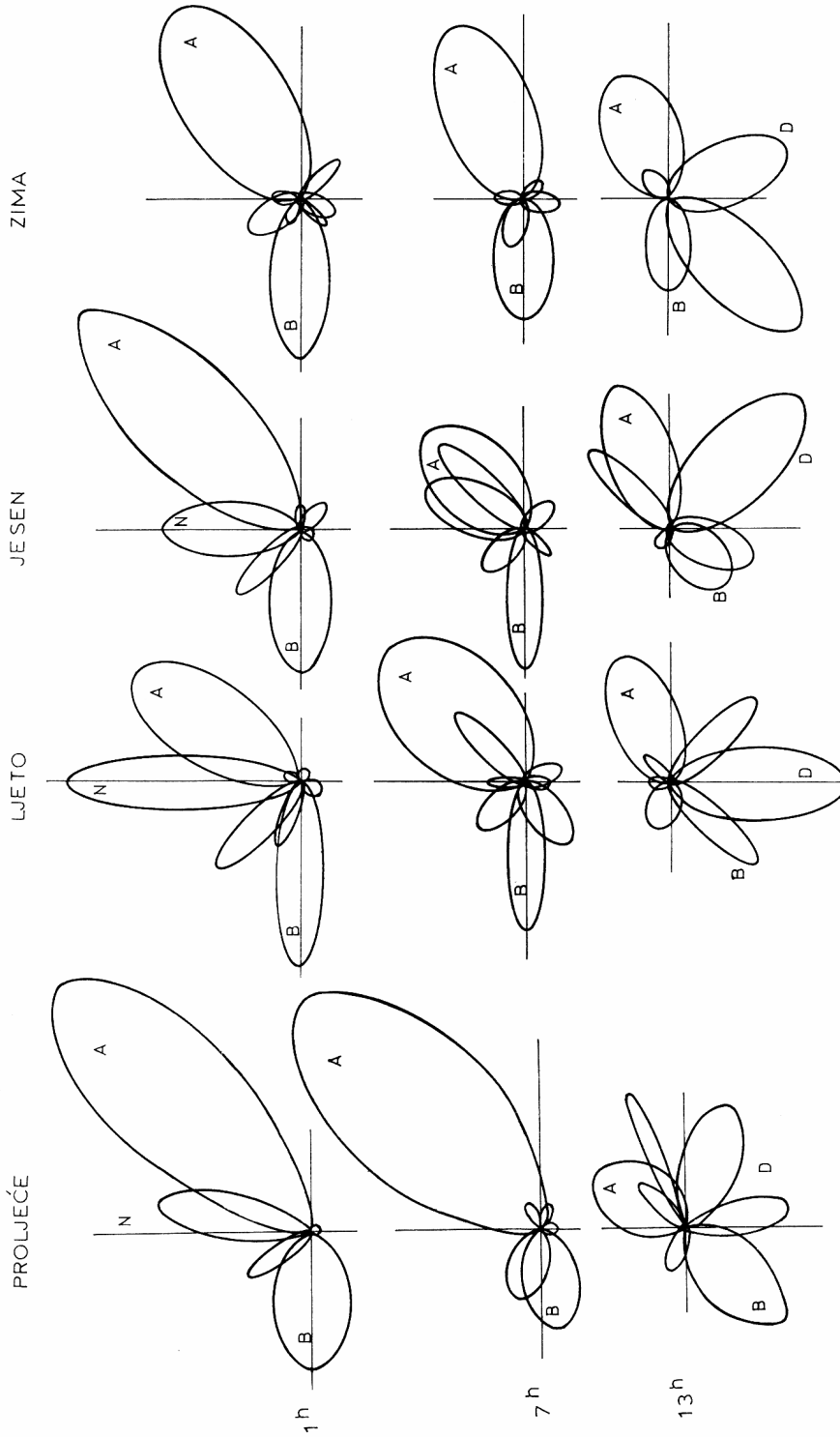
Slika 29. Osnovni kolektivni za tri dnevna termina i po godišnjim dobima, Zagreb-Grič 1956-60.
