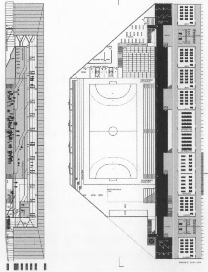
Slika 1a. Tlocrt prizemlja i presjek, I. nagrada
