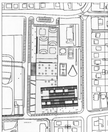
Slika 3. Situacija, II. nagrada
