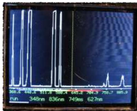
Slika 2. LCD ekran izrađenog spektrometar (na slici spektar žarulje za vrijeme perioda zagrijavanja)
