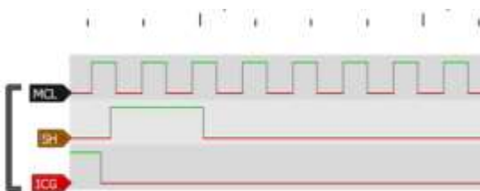
Slika 6. Inicijalizacija CCD senzora
