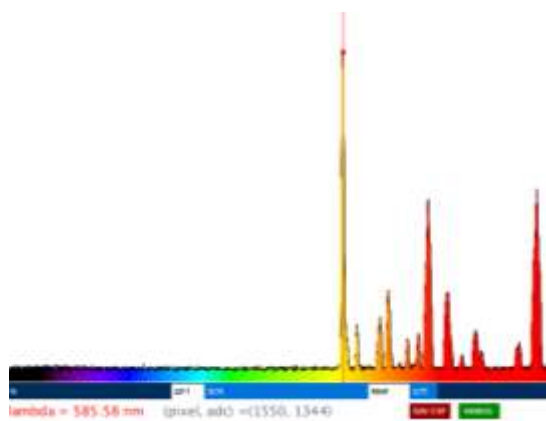
Slika 18. spektar neonske žarulje (tinjalice)
