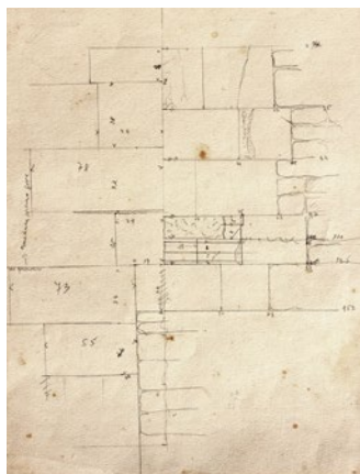
5. Grga Oštrić: arhitektonski crtež dijela južnoga zida – dilatacija između zida iz 12. i 13. stoljeća (Konzervatorski ured u Zadru)
