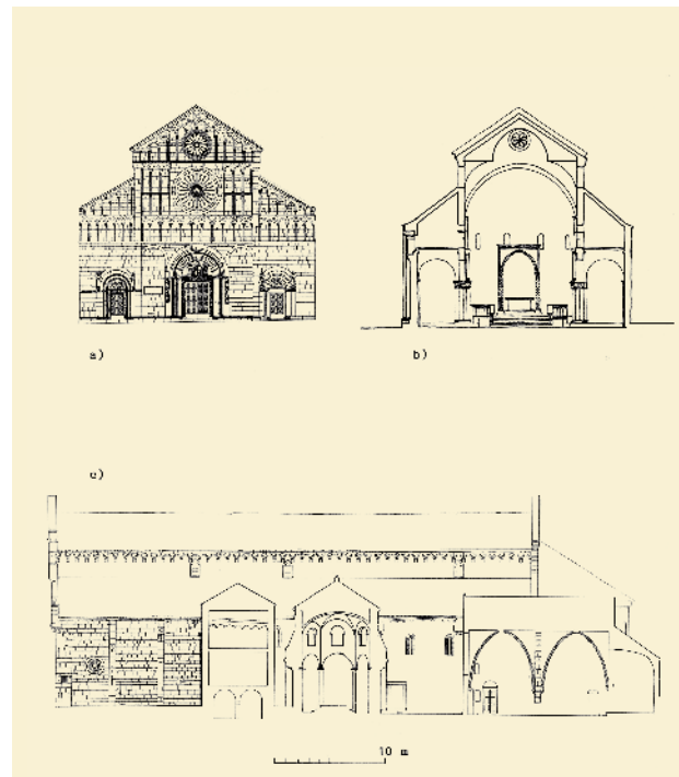
4. Nacrti katedrale: a) pročelje u 14. stoljeću, b) poprečni presjek u 15. stoljeću, c) južni zid i uzdužni presjek kroz krstionicu i sakristiju (preuzeto iz: P. Vežić, 2013.)
