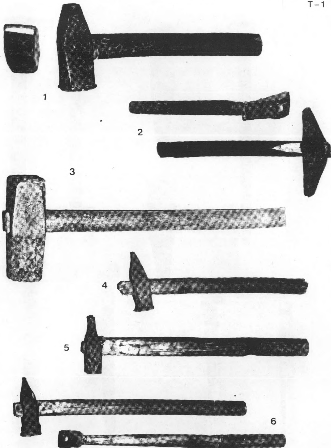
ABLA I - 1. Foršlag hamer (kladivec, prvi čekić), 2. Klepač za kosu, 3. Krajc hamer (križni čekić), 4. Pajser (za bilježenje luknjica na potkovi), Pajser, probojac, šlisdorlin (za duguljaste luknje), 6. Firkant (za probijanje okruglih luknji)
