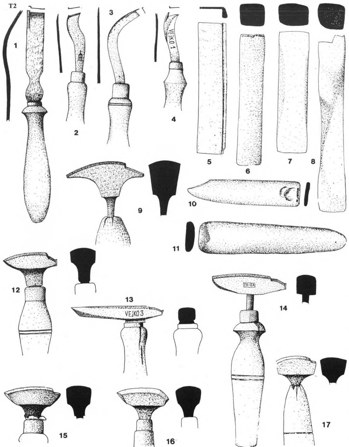
T 2 - 1 - Abnemer, oduzimač za branzil na ramu, 2, 3, 14 - Abnemer, oduzimač, 5 - ciklin, metalni strugač, 6, 7 i 8 - Gleštik, drveni za gletanje - gladenje, 9, 12, 13, 14, 15, 16 i 17 - Hampus za brenanje peta i donova, 10 i 11 - Rajpan kost za gladenje
