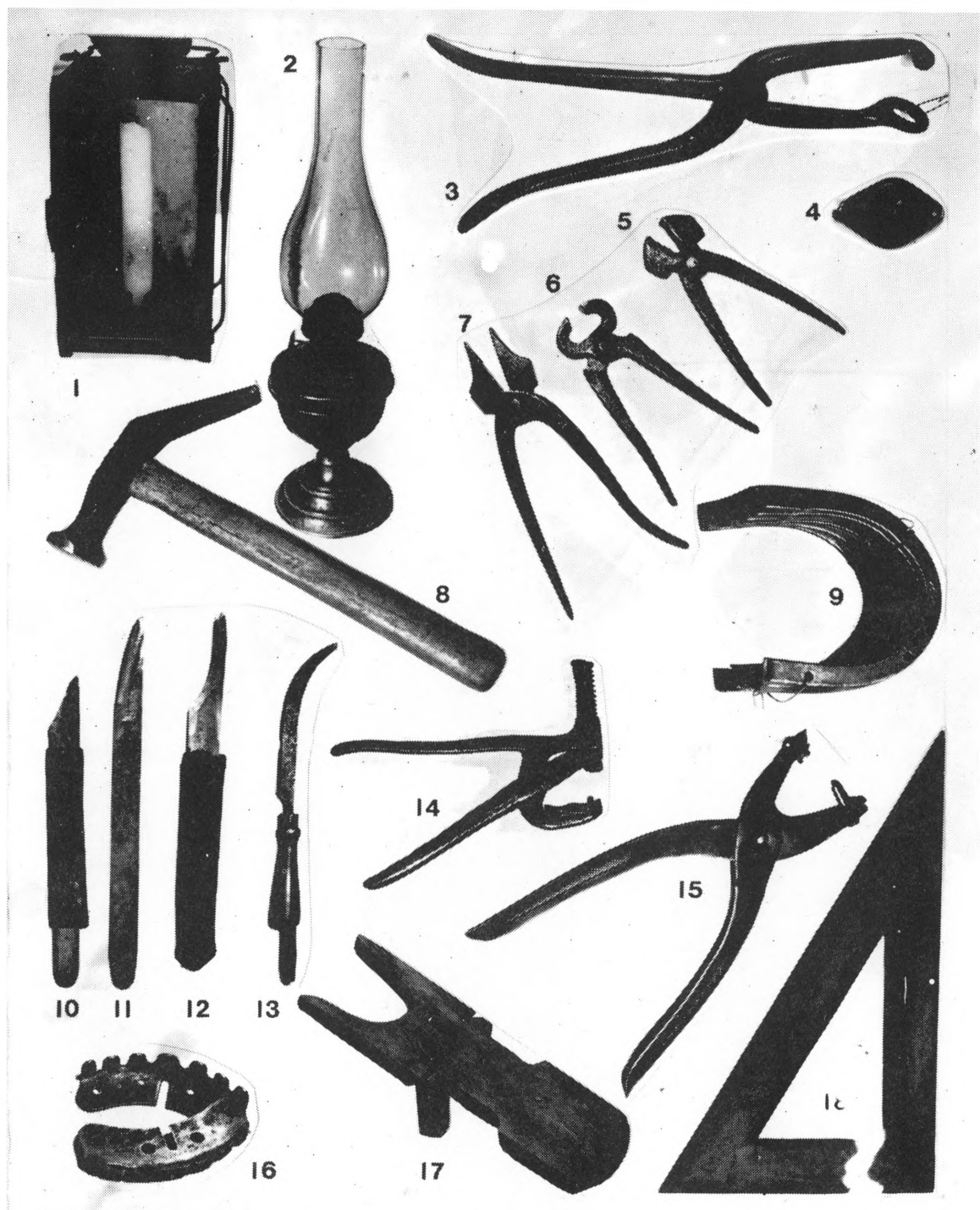
T 4 - 1 - Lampaš, 2 - Lampa petrolejka, 3 - Kliješta za natezanje kurjih očiju, 4 - Sprava za nabijanje hakni, 5 - Falcange, kliješta za cvikanje, natezanje, obrtelja za kalup, obična, 6 - Pajscange, kliješta za vadenje čavli, 7 - Falcange, kliješta za cvikanje, natezanje, 8 - Susterski čekić, 9 - Potkova, 10 i 11 - Knajp, nož za krojenje, 12 - Silf nož, 13 - Nož za obrezivanje troter peta, 14 i 15 Mašina za lohanje - bušenje, 16 - Spicplehi za bakandže, 17 - Sluga, hlapec, izuvač za čizme, 18 - Trokut za geometriju
