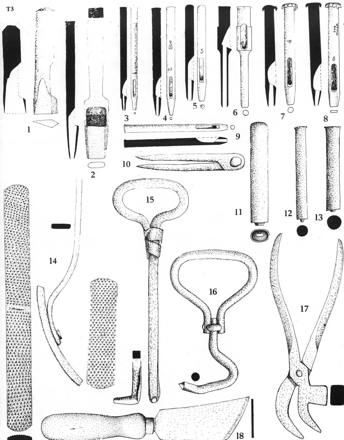
T 3 - 1 i 2 - Lohajzl, probijač za izradu ukrasnih dijelova, 3, 4, 5, 6, 7, 8 i 9 - Lohajzli za izradu rupa, 10 - cirkl, cirklin, šestar, 11, 12 i 13 - Steel za pribijanje ringle, rinčica, 14 - Holc rašpa, ravna za rašpanje klinaca i kožnih donova, 15 i 16 - Lastciger za izvlačenje kalupa, 17 - Špi-cange, klijeste za cvikanje spice, 18 - Čizmarski nož za rezanje donova
