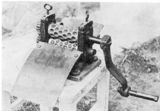
Naprava za proizvodnju bombona (Kolarić)
