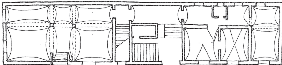
Sl. 3. Kuća Pirling, tlocrt prizemlja
