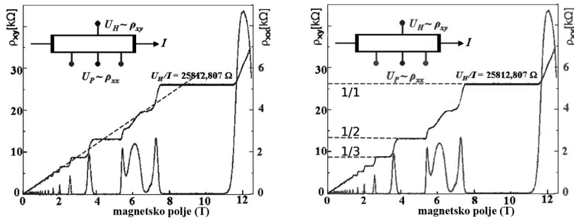
Slika 8. Rezultati Klitzingovih mjerenja Hallovog efekta za (2D) elektronski plin. Crtkana linija na lijevoj strani pokazuje očekivano ponašanje koje odudara od izmjenjenog, dok crtane linije na desnoj strani indiciraju visinu stepenica. Prikaz rezultata je preuzet iz rada [6].
