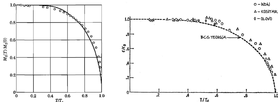
Slika 3. Na lijevoj strani prikazana je magnetizacija nikla kao funkcija temperature [1], a na desnoj temperatura ovisnost energijskog procjepa u supravodljivoj fazi za In, Sn i Pb [2].
