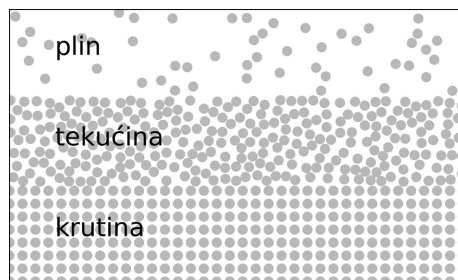
Slika 2. Agregatna stanja.
