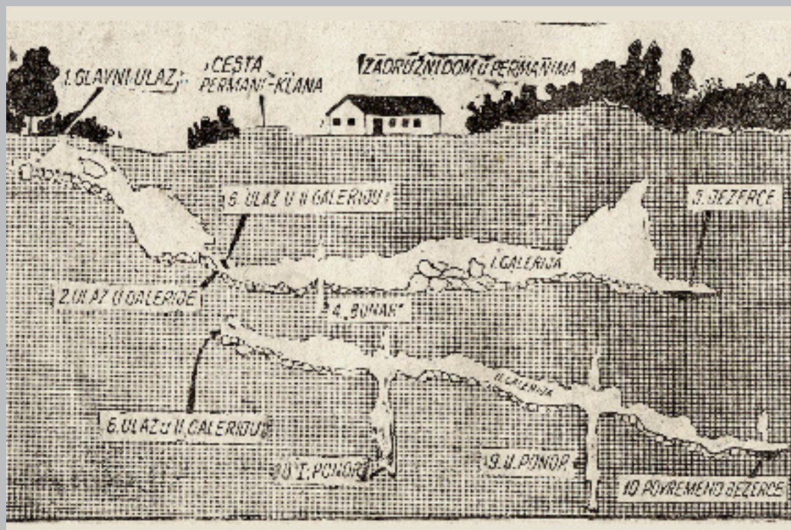
Preslika nacrtu Jame na Puharevom iz VUS-a od 13. 07.1960, str. 6.
