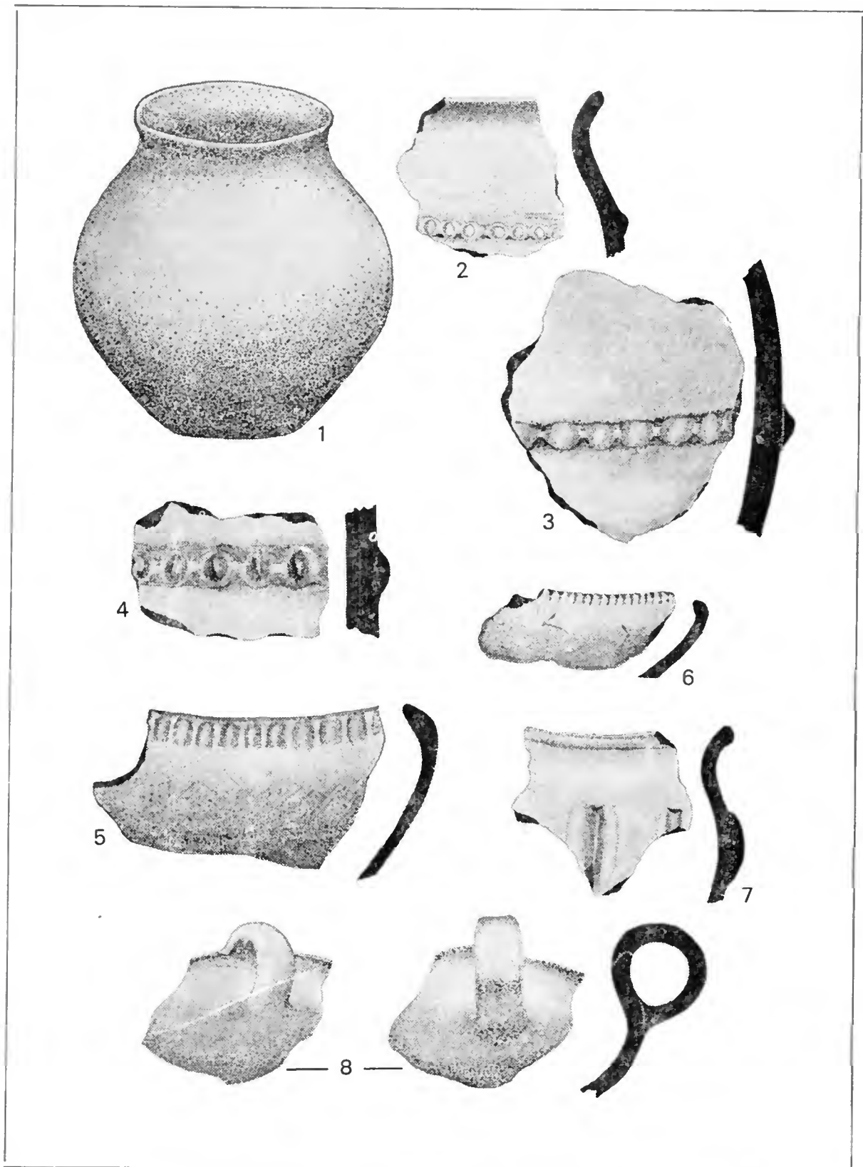
T. I Kamenj Vrh: 1 — 8 keramika; sve 1:3 (Crteži: B. Šimek) Kamenj vrh: 1 — 8 Ton; alles 1:3 (Zeichnungen: B. Šimek)
