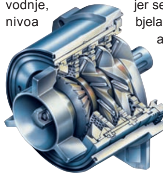
◀ INOTEC - rezni sustav s 3 rezne glave / kombinacije reznih pločica (4 nivoa usitnjavanja)
