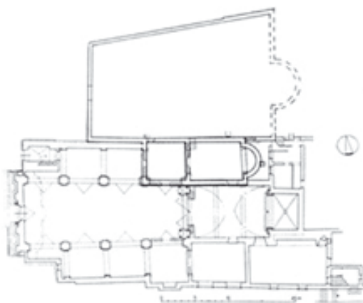
Crtež 1. Izradio Ivo Štambuk 1992. za Nikšu Petrića, s ucrtanom crkvom pod kapelom sv. Prospera u hvarskoj katedrali.
