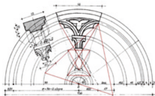
Sl. 9. Proporcije rozete gotičke katedrale. Crtao Ivo Štambuk.
