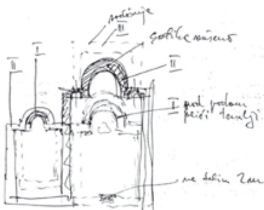
Crtež 3. Nalaz u prezbitariju hvarske katedrale izrađen kada se kopalo 1991. za izradu biskupske grobnice i temelja za novi oltar. Skicirao Ivo Štambuk.
