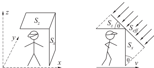
Slika 1. Pojednostavnjena geometrijska razmatranja za izvod ovisnosti pokisnuća.
