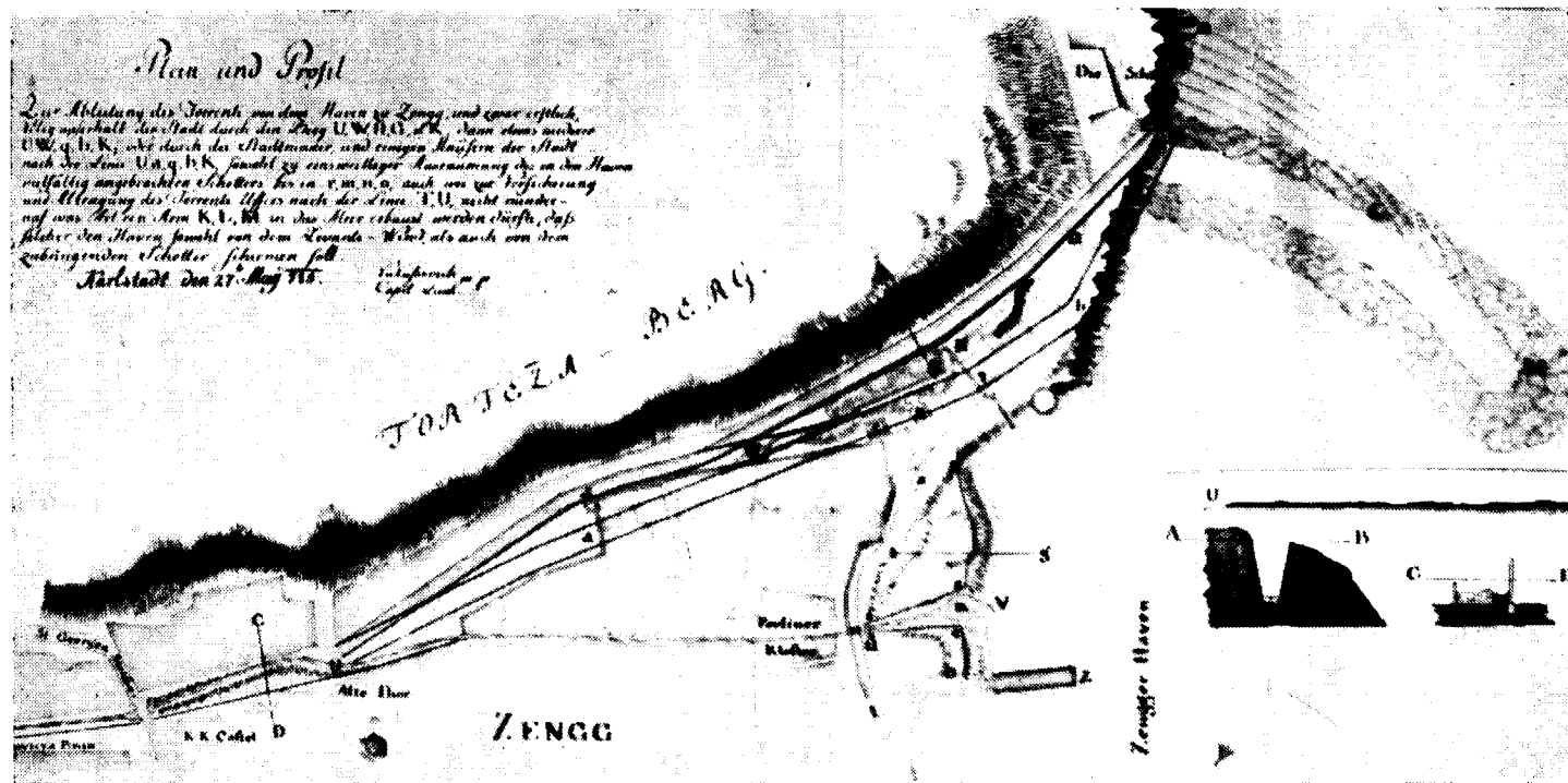
Sl. 11. — Plan i profil (Copia) odvođenja Potoka od senjske luke, i to u prvom redu potpuno izvan grada kroz brijeg U, W, H, G, i K, onda nešto niže U, W, g, h, K, ili kroz gradski zid i gradske kuće prema liniji U, a, q, h, K, — kao i privremeno čišćenje (jaruženje) u luci nagomilanog šljunka sve do r, m, n, o, nadalje osiguranja i snižavanja obale Potoka prema liniji T, U, te na koji način bi se sagradio u moru lučki nasip (molo) K, L, M da zaštićuje luku od vjetra levantinca kao i od nanosa šljunka.
