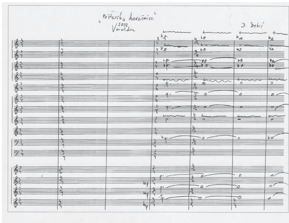
Slika 7. Fragment koračnice
