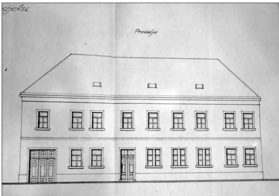
Slika 4: Nacrtna dogradnja
