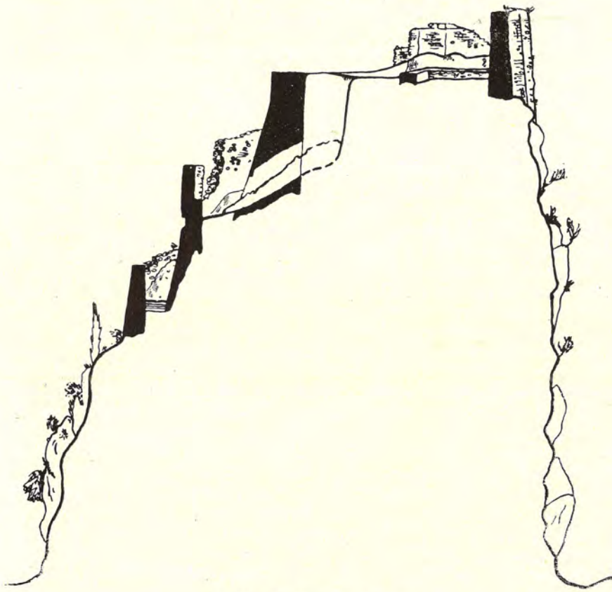
Grad Soko. Poprečni presjek
