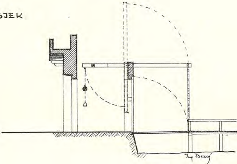
Rekonstrukcija »Vrata zamirja« ili »Kopnenih vrata«
