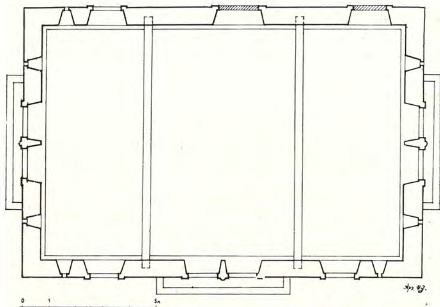
1. Zdravković: Tlocrt drugog kata Bujovićeve palače
