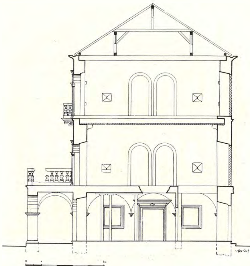
1. Zdravković: Bujovićeva palača (presjek)
