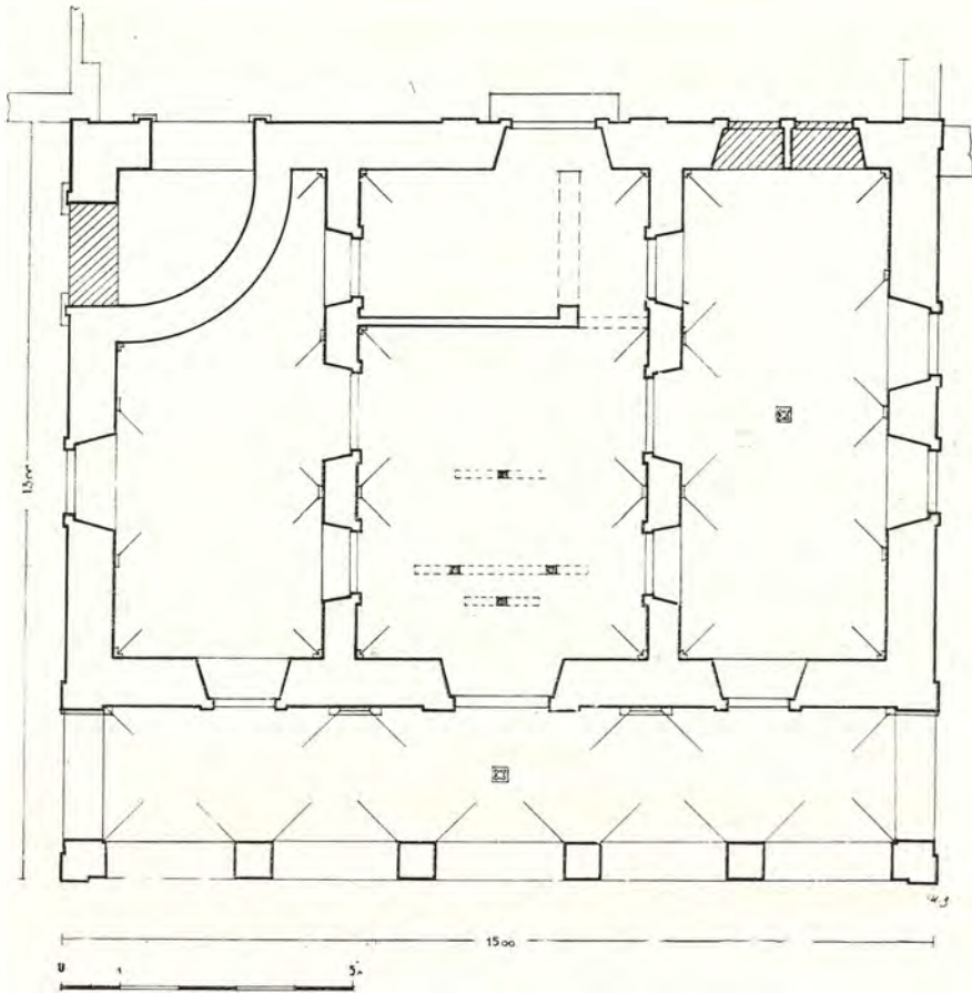
I. Zdravković: Tlocrt prizemlja Bujovićeve palače
