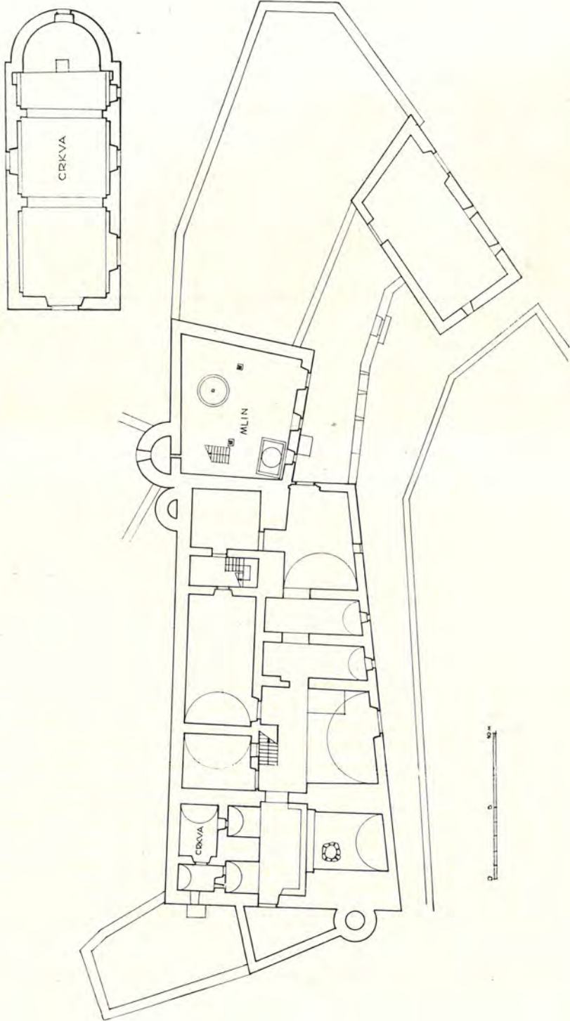
D. Živanović: Tlocrt prizemlja manastira Podostroga
