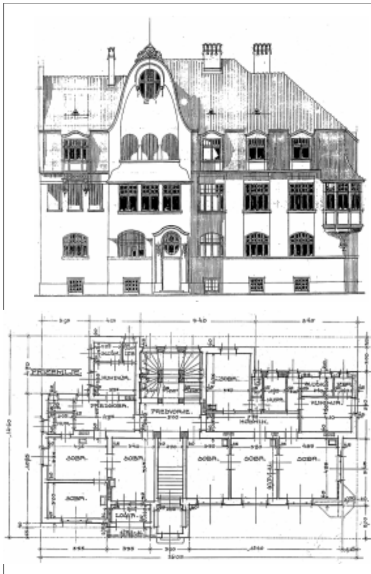
SL. 5. Kuća Marković, Nazorova 20 (1910/1911.)
