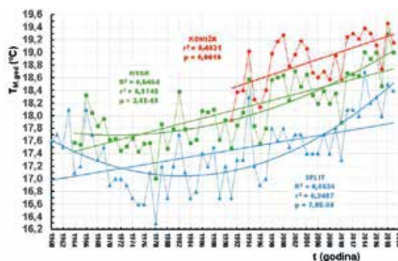
Slika 2: Nizovi srednjih godišnjih temperatura površine mora, T_{Mpr} opaženi na tri analizirane postaje: (1) Split (1960. - 2019.; plava boja); (2) Hvar (1964. - 2019.; zelena boja); (3) Komiža (1991. - 2019.; crvena boja)
