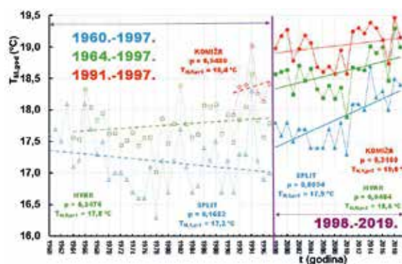
Slika 3: Podnizovi srednjih godišnjih temperatura površine mora, T_{Mpr} opaženi na tri analizirane postaje definirani RAPS metodom: (1) Split (plava boja); (2) Hvar (zelena boja); (3) Komiža (crvena boja)
