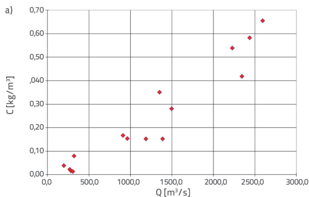
Slika 8. a) Odnos koncentracije mase suspendiranog nanosa i protoka, b) Granulometrijske krivulje za suspendirani nanos (1) i vučeni nanos (2)
