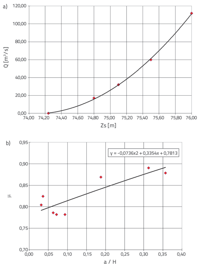
Slika 5. a) Odnos protoka ( Q ) i vodostaja ( Z_s ) za tok vode preko klapni zapornice, b) Koeficijent protoka ( \mu ) ovisno o položaju segmentne zapornice (a-otvor zapornice, H-dubina u uzvodnom dijelu)
