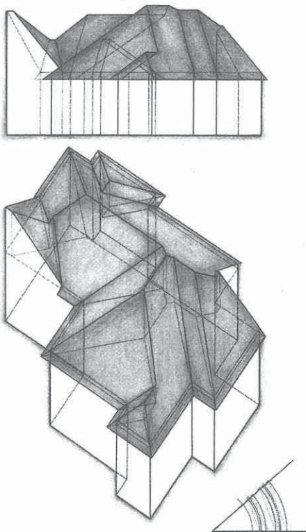
4. Krovšte, nacrt i aksonometrija
