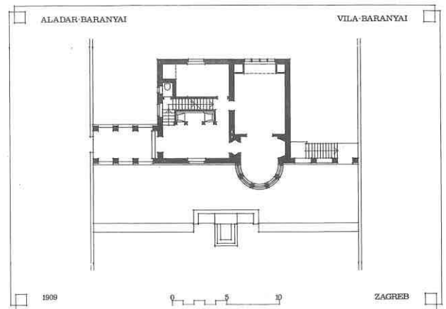
Prva vila Baranyai na Tuškancu, 1909.-10. Tlocrt prema urudžbenom planu, precrct arh. grade AL.
