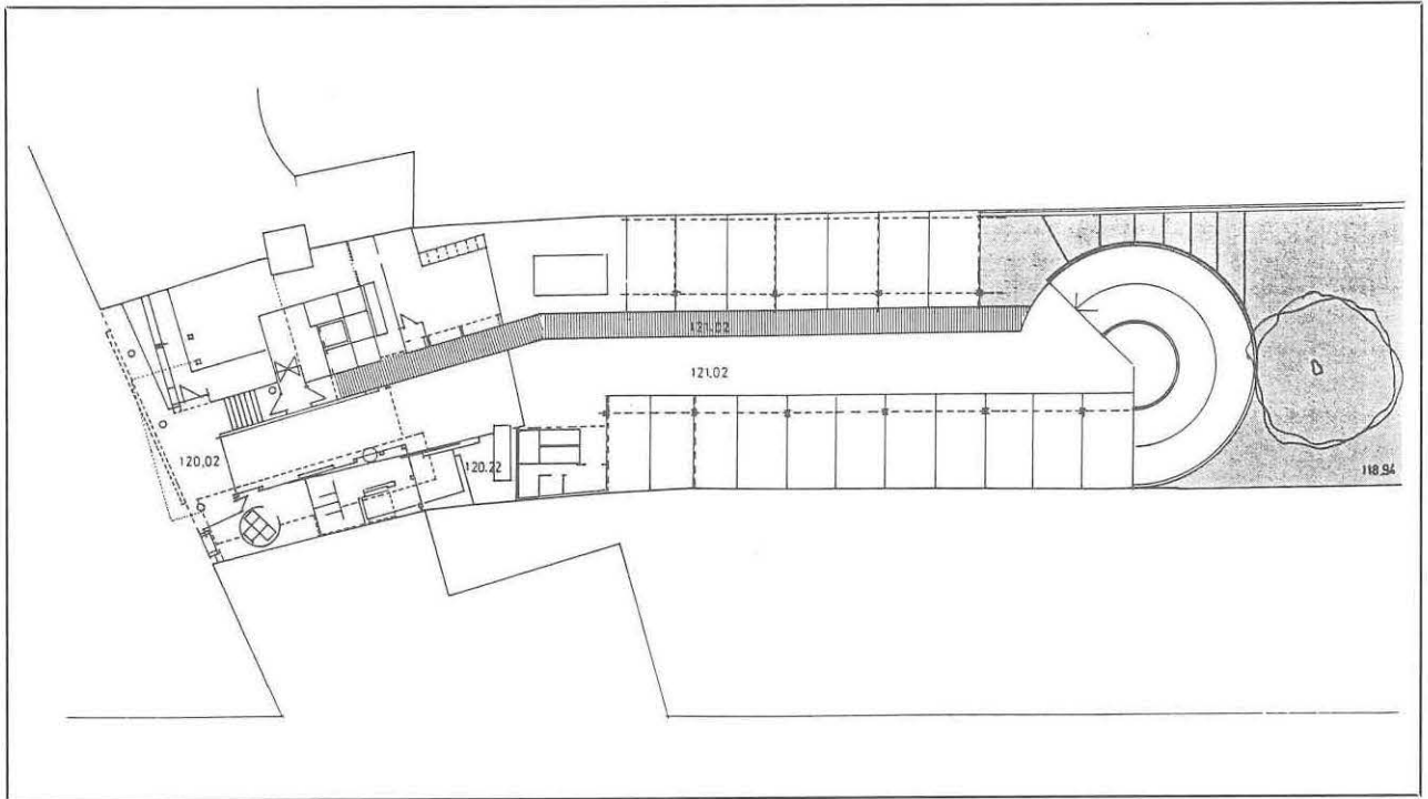
S. F. & V. M. Projekt interpolacije stambeno-poslovnog objekta, Petrinjska 9, Zagreb, 1992.
