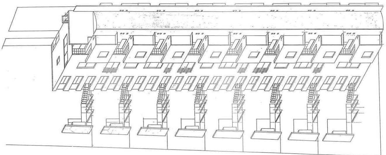
S. F. & V. M. Projekt stambenog niza na Kajzerici, Zagreb, 1989.
