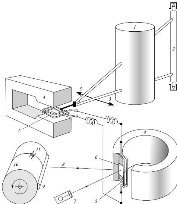
Slika 2. Seizmograf – 1. fizikalno njihalo, 2. osovina, 3. smjer njihanja, 4. magnet, 5. indukcijski namotaj, 6. zrcalo, 7. izvor svjetlosti, 8. odbijena zraka, 9. leća, 10. kronograf s fotopapirom, 11. zapis. Izvor: Hrvatska enciklopedija
