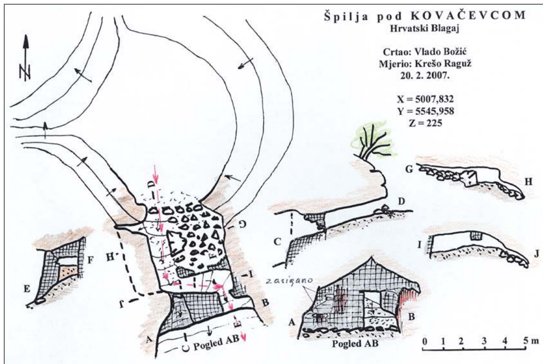
Tlocrt utvrde Špilje pod Kovačevcom (strelica pokazuje smjer kretanja)
