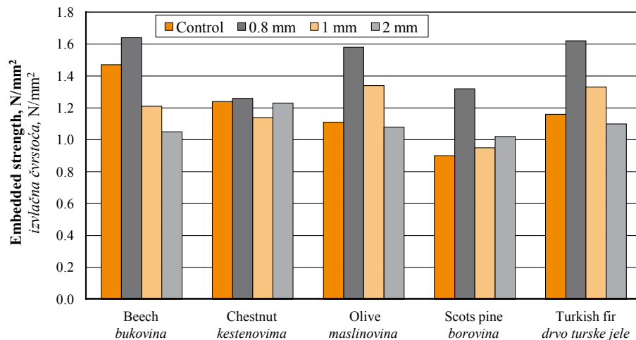
Figure 6 Effect of interactions of thickness of PVC edge banding and wooden dowel species on embedded strength Slika 6. Utjecaj interakcije debljine PVC rubne trake i vrste drva moždanika na izvlačnu čvrstoću
